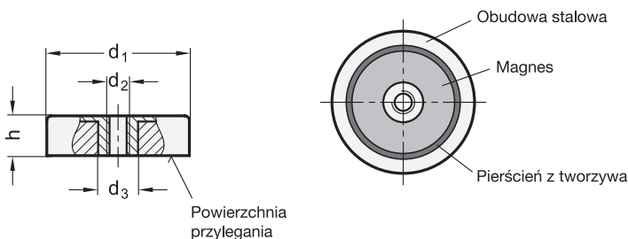
Widok od strony przylegania
